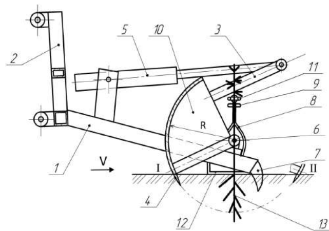
Қазиш-трансплантация бўлини маси прототипининг умумий кўриниши
