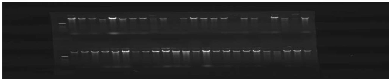
1-rasm. 0.9% li agaroz gelidagi g'o'za namunalariining elektroforegrammasi.
