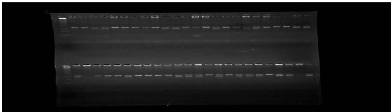
2-rasm. BNL-3436 DNK markeri bilan olib borilgan PZR mahsulotlarining elektroferogrammasi.
