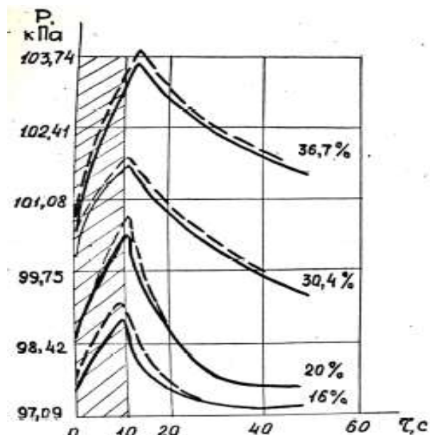
Расм-4. УЮЧ қиздиришдаги капилляр босимининг ўзгариши P_{\text{свч}} = 0,36 \text{ кВт} , \tau = 50 \text{ сек} .
