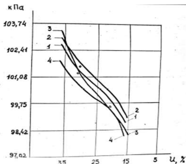
Расм-5. Мева ва сабзавотларни УЮЧ қиздиришдаги капилляр босимининг намлигига боғлиқлиги P_{\text{свч}} = 0,45 \text{ кВт} , \tau = 30 \text{ сек} .
