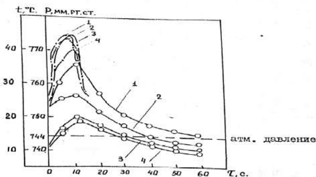
Расм-3. УЮЧ қиздиришда мева ва сабзавотлар капилляр босимининг ўзгариши. P_{\text{свч}} = 0,45 \text{ кВт} , \tau = 30 \text{ сек} .
